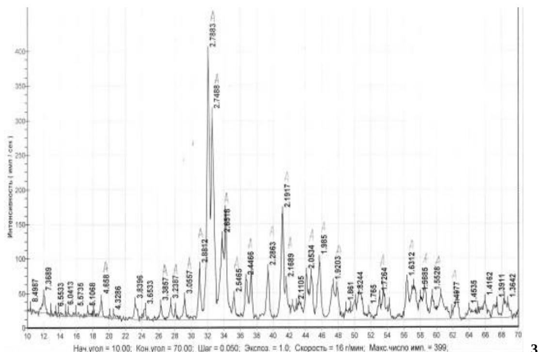
Сурет 15- 1300 °С температурада күйдірілген клинкерлердің ретгенограммалары
