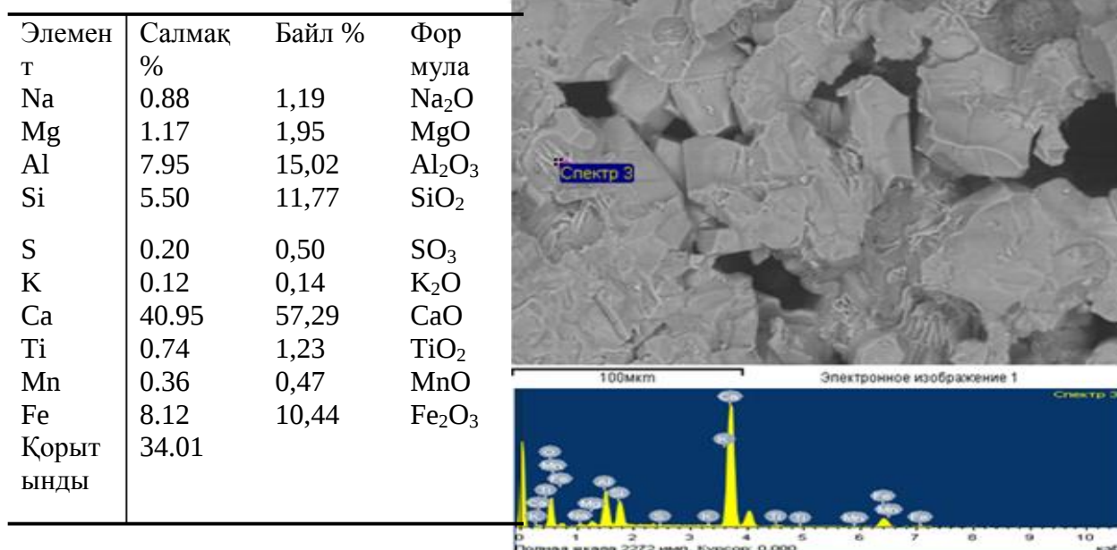
Сурет 12 - 1350 °C температурада күйдірілген № 4 клинкердің құрылымы және құрамы C 4 AF, электронды-микроскопиялық талдау деректері бойынша
