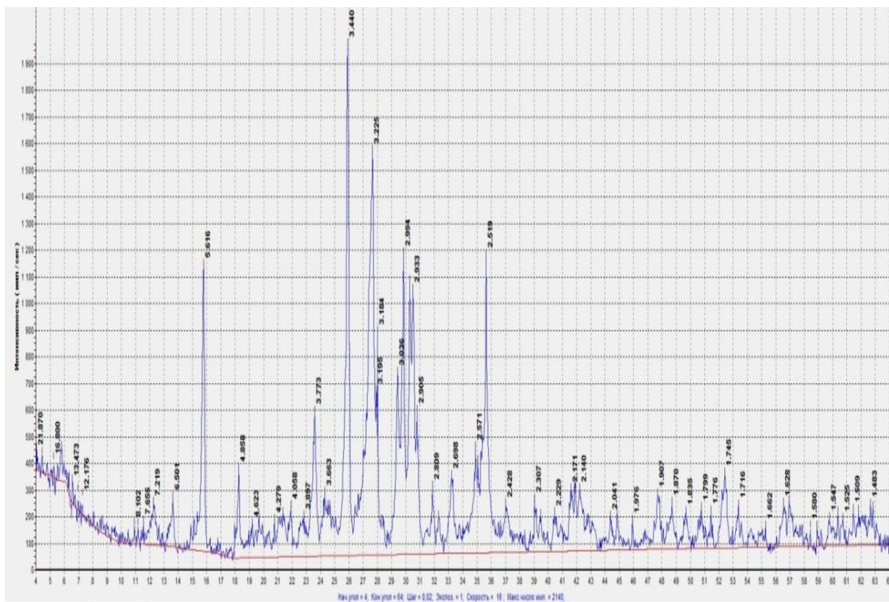
Сурет 4 – «Южполиметалл» АҚ зауытының қорғасын шлағының рентгенограммасы
