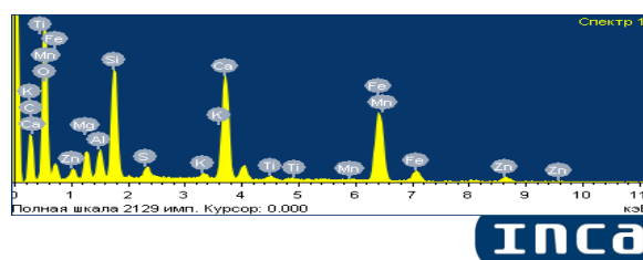
Сурет 1 – Ащысай металлургия зауытының мырыш кендерін вельцилеу клинкерінің растрлық электронды-микроскопиялық талдауы
