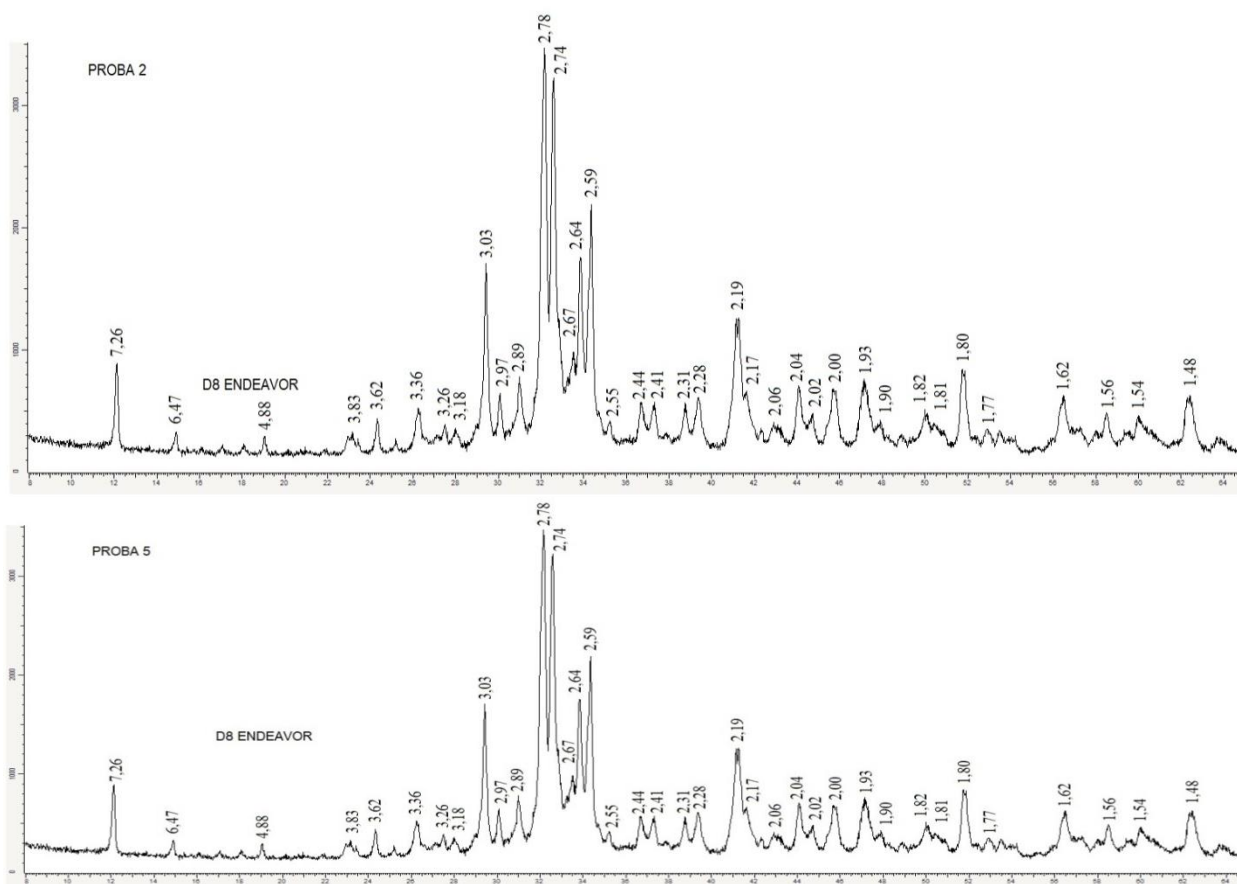
Сурет 13 – «Ащысай клинkerімен» әктас - лесс шикізат қоспасы негізінде аз энергияны қажет ететін клинkerлердің № 6 және № 9 рентгенограммалары
