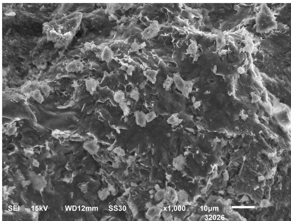
Сурет 8 – «Әктас қалдықтары + лесс + қорғасын шлағы» дәстүрлі емес шикізатынан алынған клинкердің сынықтарынан алынған микрофотографиясы
