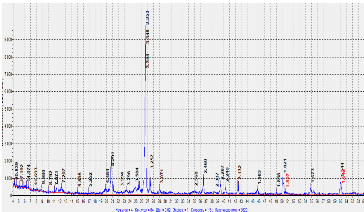
Сурет 6 – Ленгер шахталарының көмір өндіру қалдықтарының рентгенограммасы
